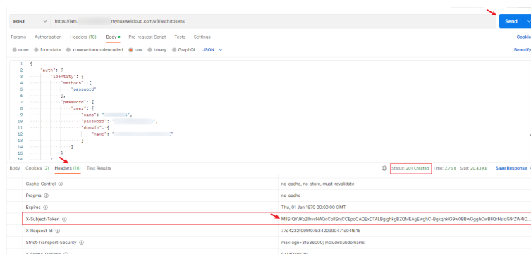
图 2-5 获取 Token
